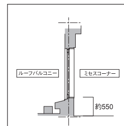
B—B' 断面図 S=1:100
