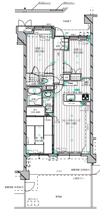
Hg type全体図 S=1:190
