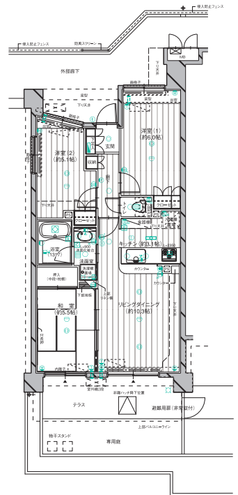
Gg type全体図 S=1:190
