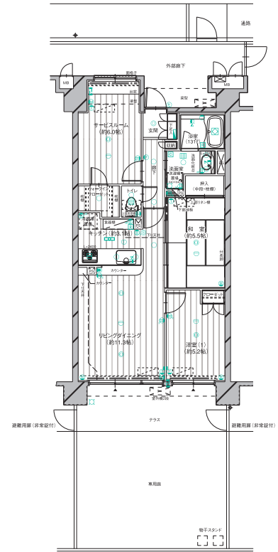
Eg type全体図 S=1:190
