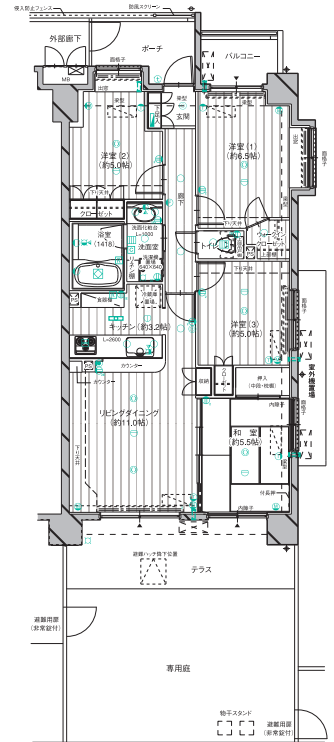
A'g type全体図 S=1:190
