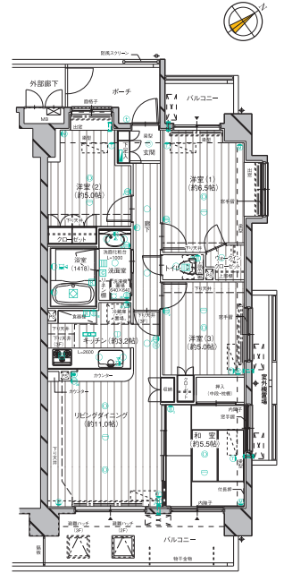
A type全体図 S=1:190
