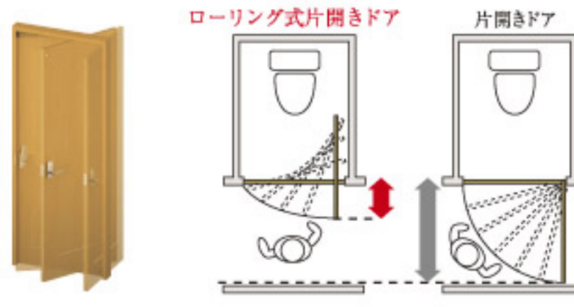
【33-3】ローリング式片開きドア(DAIKEN)
